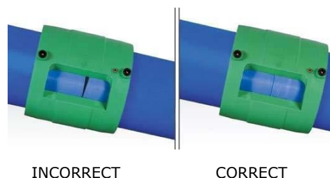
Figure 12 - Pour un processus optimal de soudure, les tubes doivent être placés en bout à bout dans le manchon. La profondeur minimale d'introduction doit toujours être respectée
