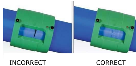
Figure 12 - Pour un processus optimal de soudure, les tubes doivent être placés en bout à bout dans le manchon. La profondeur minimale d'introduction doit toujours être respectée
